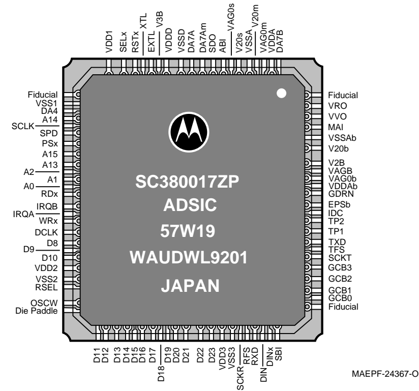
U405 - DSP
