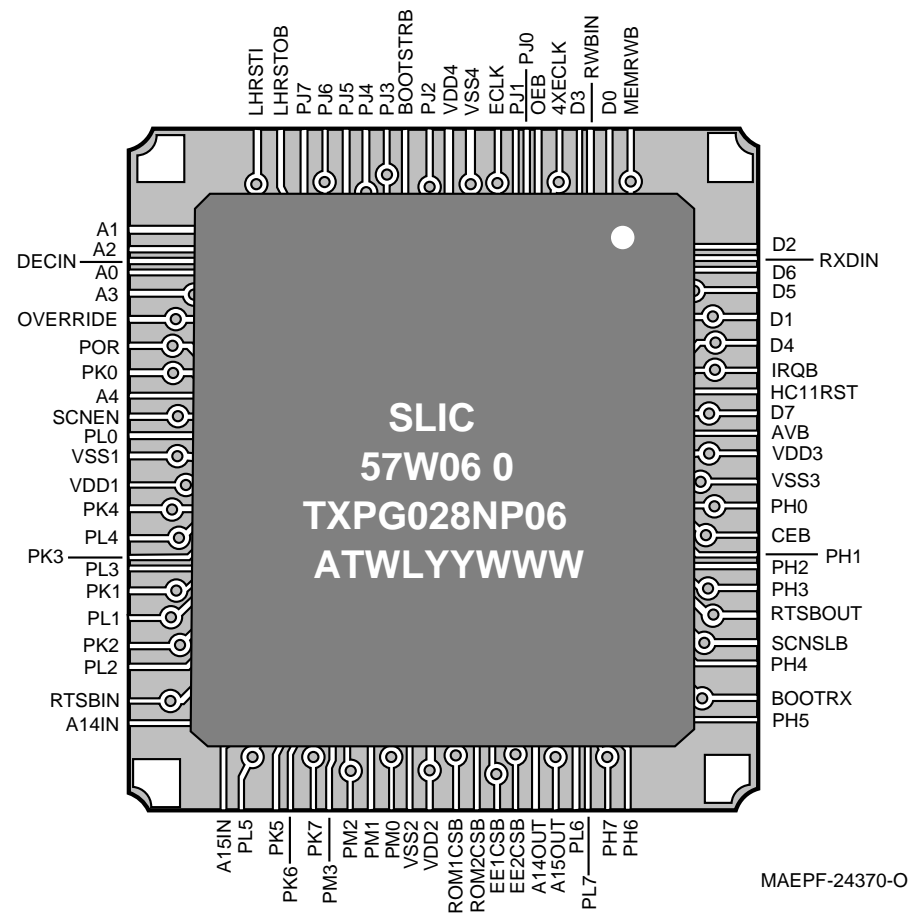
U206 - SLIC
